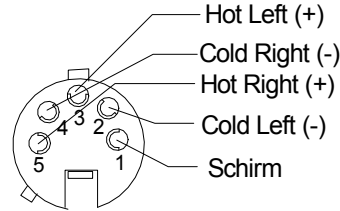
Audio Technica Mikrofon Rückansicht ( AT825 ) XLR - Female 5 Pol
