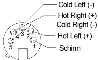
Rückansicht ( Normal ) XLR - Female 5 Pol
