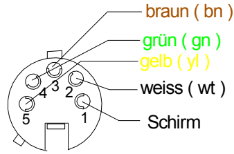
DMX-Belegung Rückansicht XLR - Female 5 Pol
