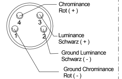
Rückansicht Y/C - S4P
