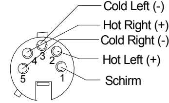
Sennheiser Mikrofon Rückansicht ( MKE 44 P ) XLR - Female 5 Pol
