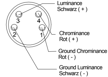
Rückansicht Y/C - S4J
